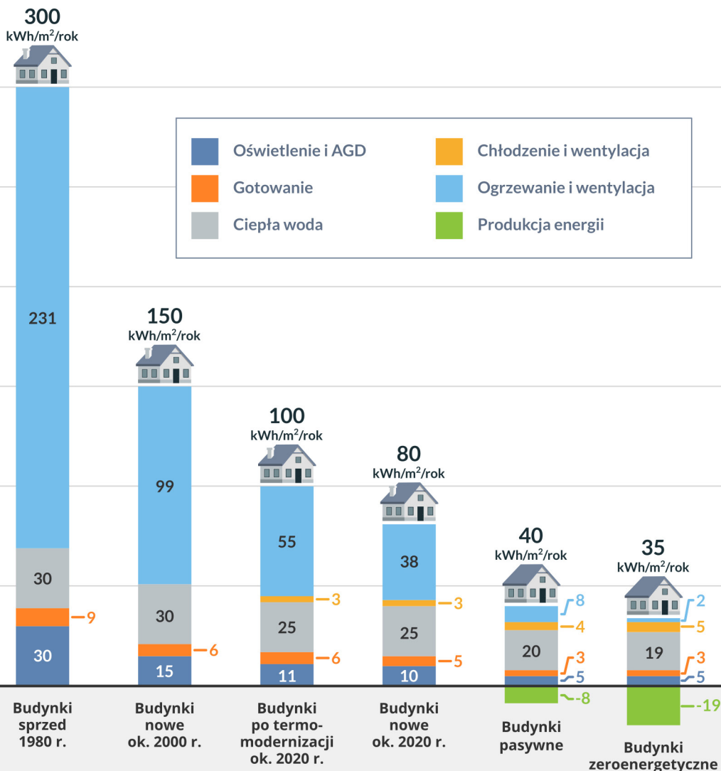
Rysunek 2: Orientacyjna struktura i zużycie energii użytkowej (kWh/m 2 /rok) w budynkach o różnym standardzie technicznym
